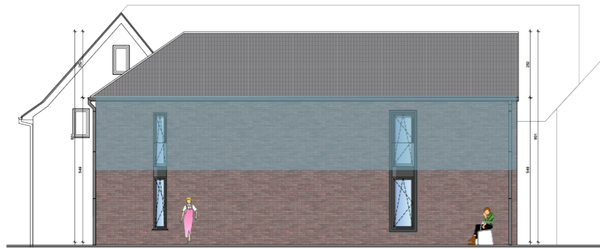
rechterzijgevel
