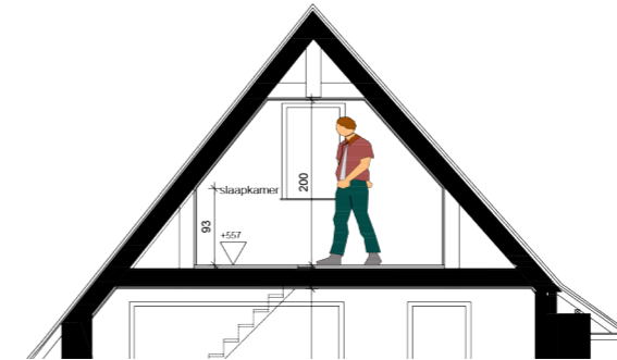
doorsnede slaapkamer
